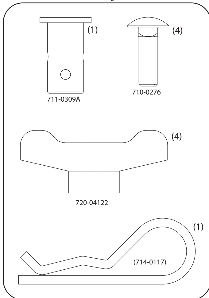
Jeu de montage 689-00328
